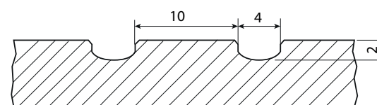
Schemat aplikacji frezowanej
