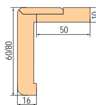
Opaska kątovej 60/80 mm z klipsem MDF za dopłatą
