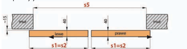
System podwójny
