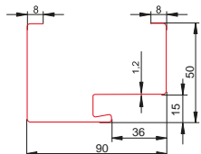
Ościeżnica stalowa z uszczelką FD-25/21B
