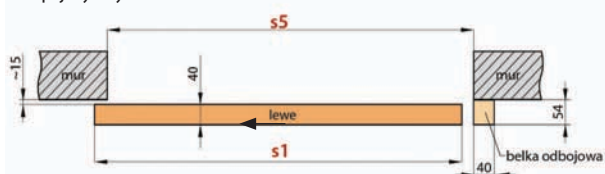
System podwójny
