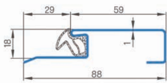
Próg stalowy.
