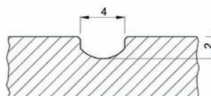
Schemat aplikacji frezowanej
