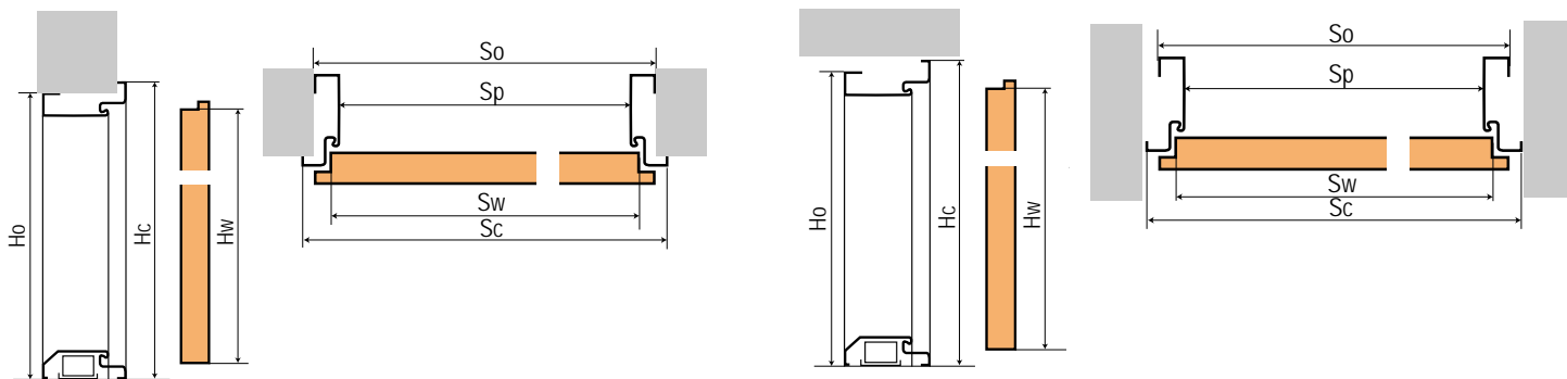
Rys. nr 2 Osadzenie ościeżnicy wewnątrz muru.
