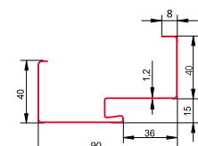
Ościeżnica stalowa z uszczelką FD-25/21C
