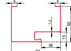
Ościeżnica stalowa z uszczelką FD-25/21B
