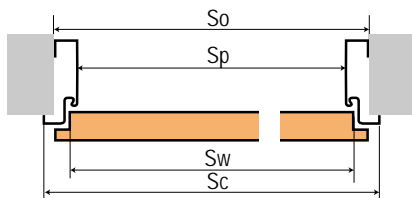
Ościeżnica stalowa z uszczelką FD-25/21C
