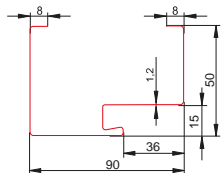
Ościeżnica stalowa z uszczelką FD-25/21B
