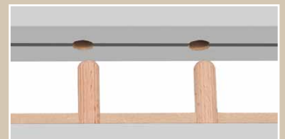
Trwałe połączenie kołkowe
