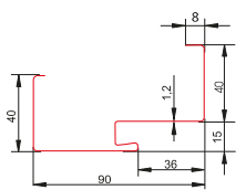
Ościeżnica stalowa z uszczelką FD-25/21C
